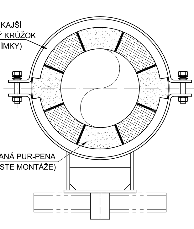
ČELNÝ POHĽAD
