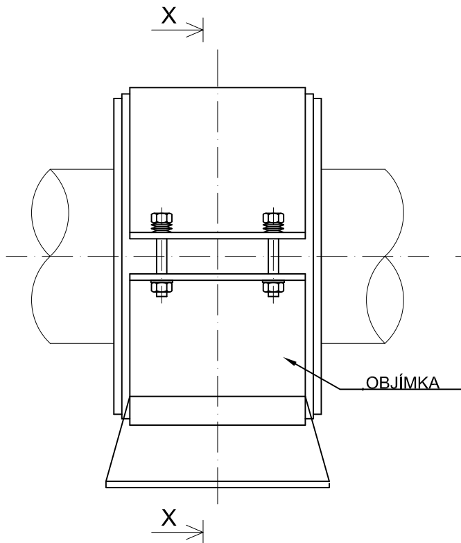
BOČNÝ POHĽAD
