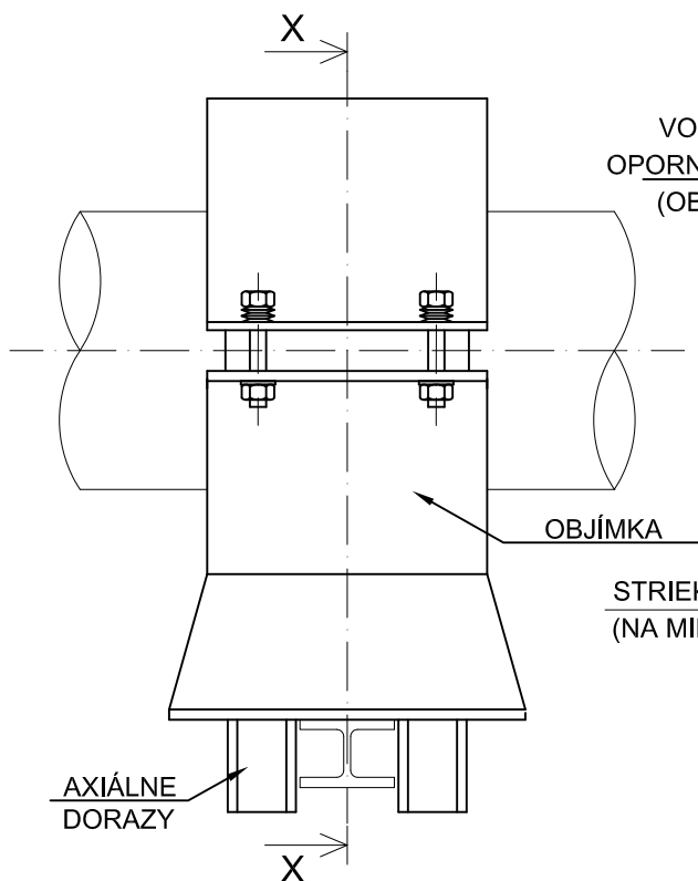
BOČNÝ POHĽAD
