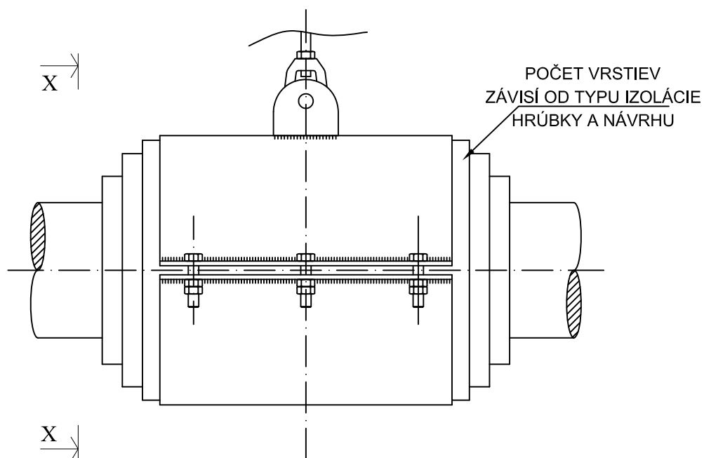
bočný pohľad
